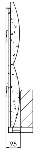
SEZIONE A-A SCALA 1 : 12
