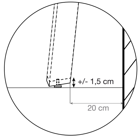
REGOLAZIONE LIVELLATORI LEVELLING FEET ADJUSTMENT
